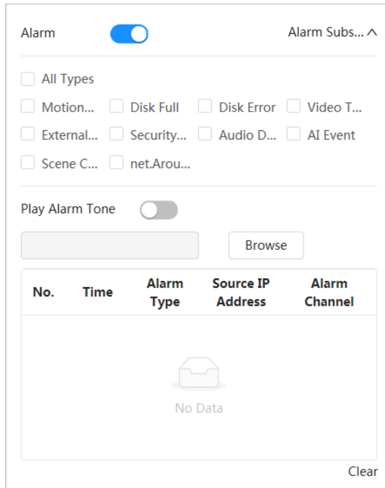
Figure 4-68 Alarm (subscription)
