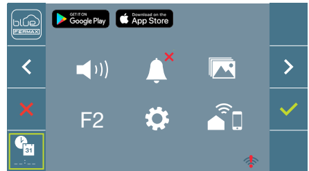
Bildschirm: BENUTZERENÜ
