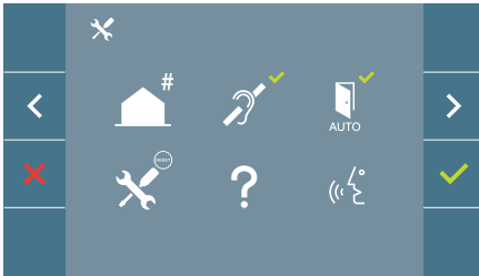
Bildschirm: ADMINISTRATORENÜ
