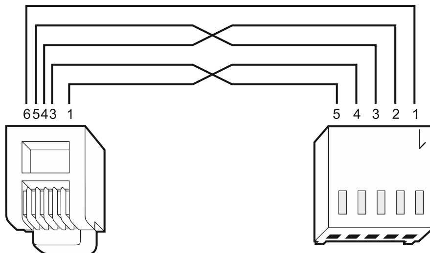
Rys. 5. Schemat kabla służącego do połączenia portów RS-232 modułu INT-GSM i centrali INTEGRA / INTEGRA Plus z gniazdem typu RJ.
