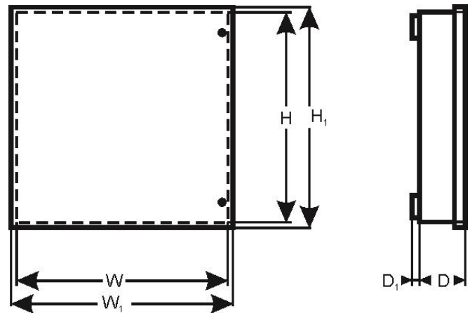
Rys.3. Widok zasilacza.
