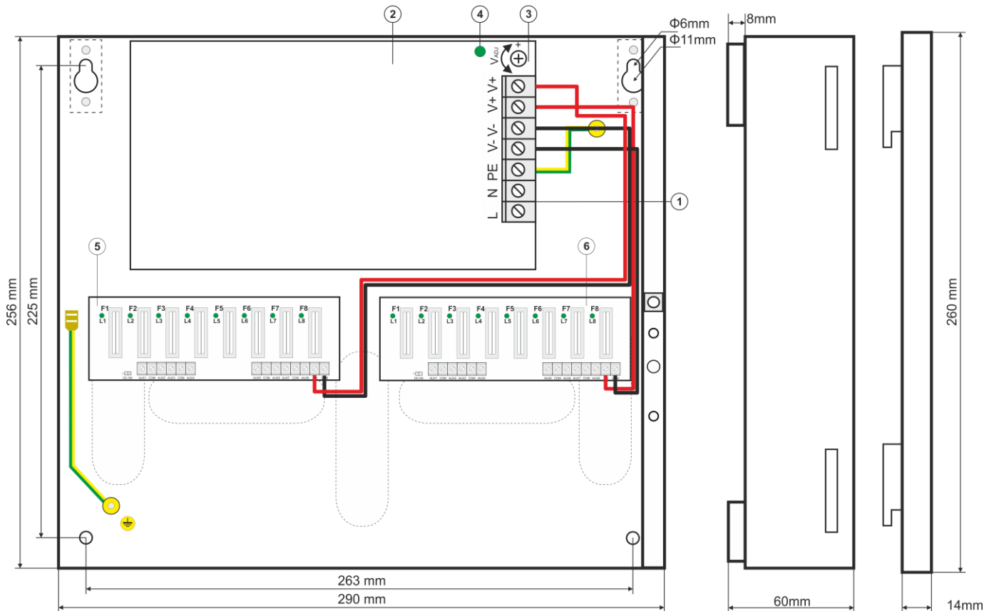
Rys.3. Widok zasilacza.
