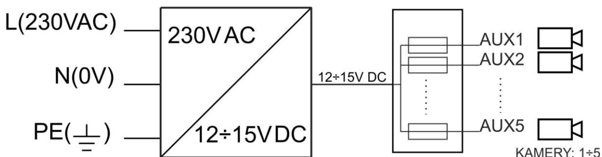
Rys.1. Schemat blokowy zasilacza.
