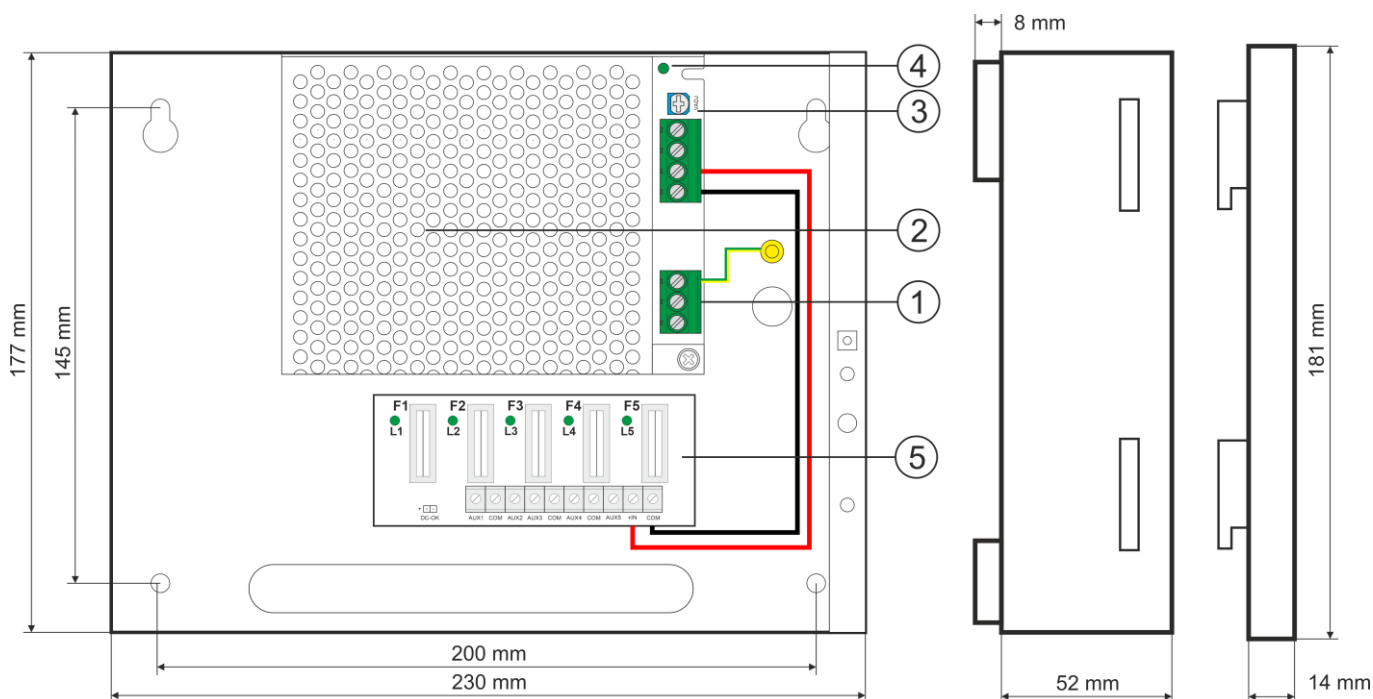
Rys.3. Widok zasilacza.
