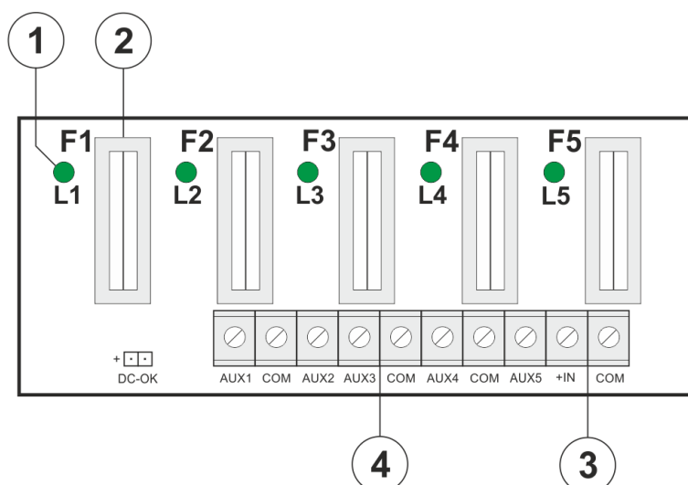
Rys. 2. Widok płyty PCB zasilacza.
