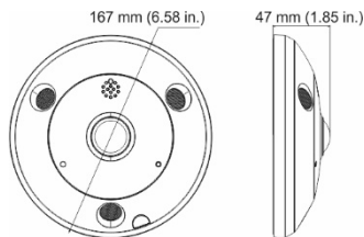
Wymiary kamery zewnętrznej:
