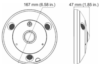
Wymiary kamery wewnętrznej:
