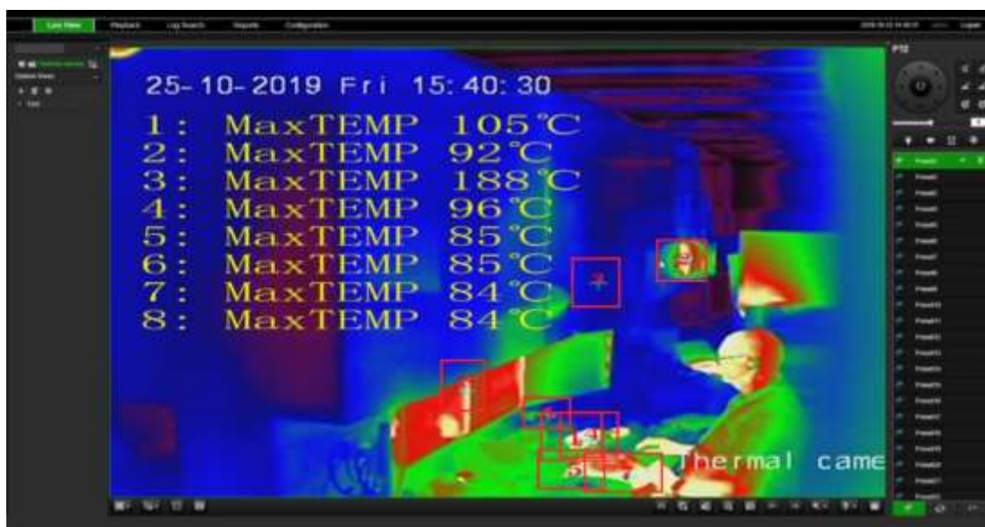
Rysunek 35: Przykładowy widok wyników działania funkcji Punkt zapłonu w oknie podglądu na żywo
