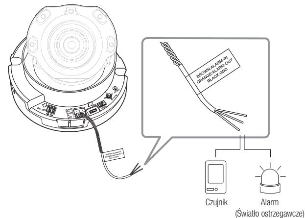
<XND-6080/6080V/6080R/6080RV/8080R/8080RV>
