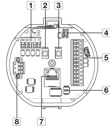
Widok podstawy instalacyjnej wewnątrz
