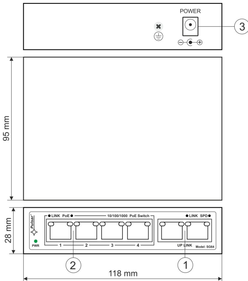
Rys. 3. Widok switch'a.
