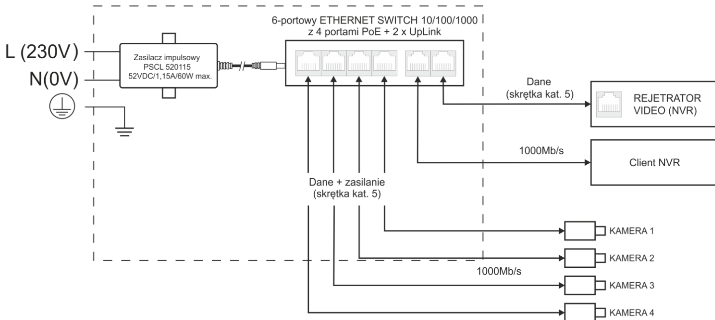
Rys. 1. Schemat blokowy.
