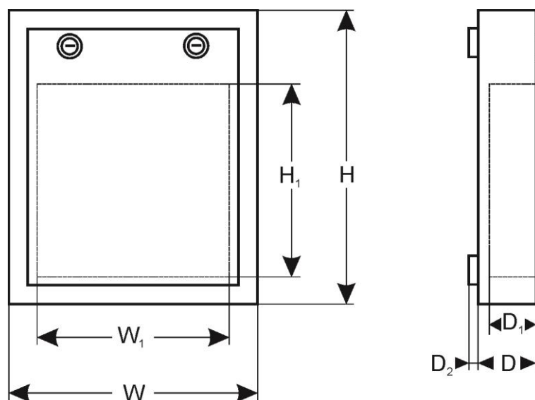
Rysunek 1. Wymiarowanie.
