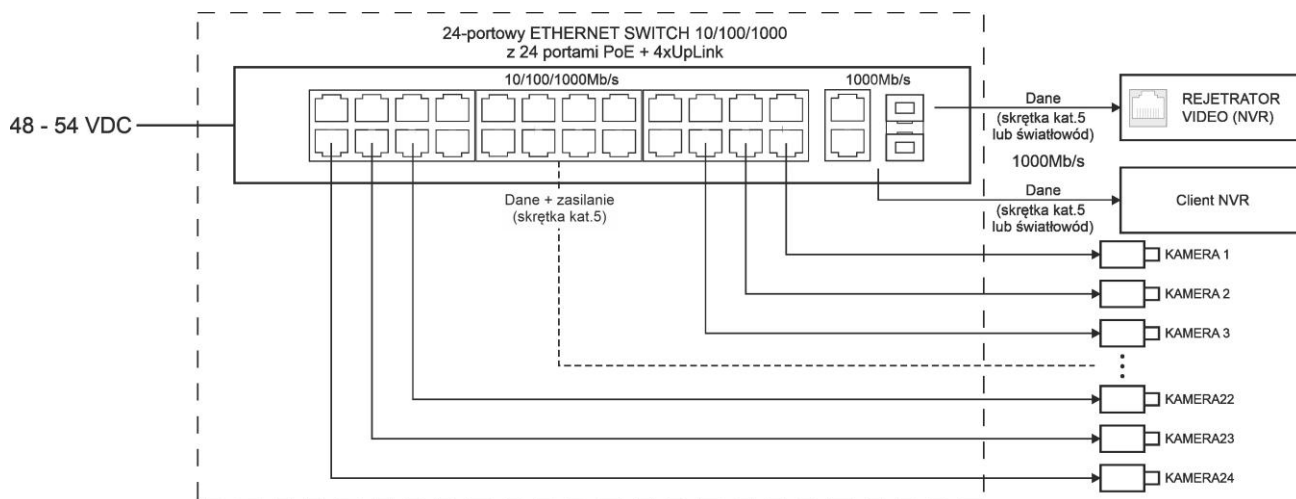
Rys. 1. Schemat blokowy.
