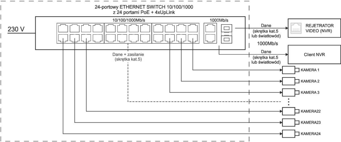
Rys. 1. Schemat blokowy.
