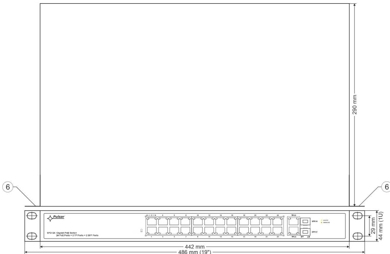
Rys. 4. Widok switch'a.
