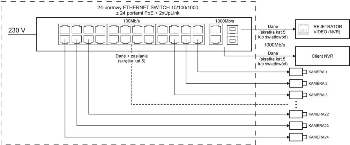
Rys. 1. Schemat blokowy.
