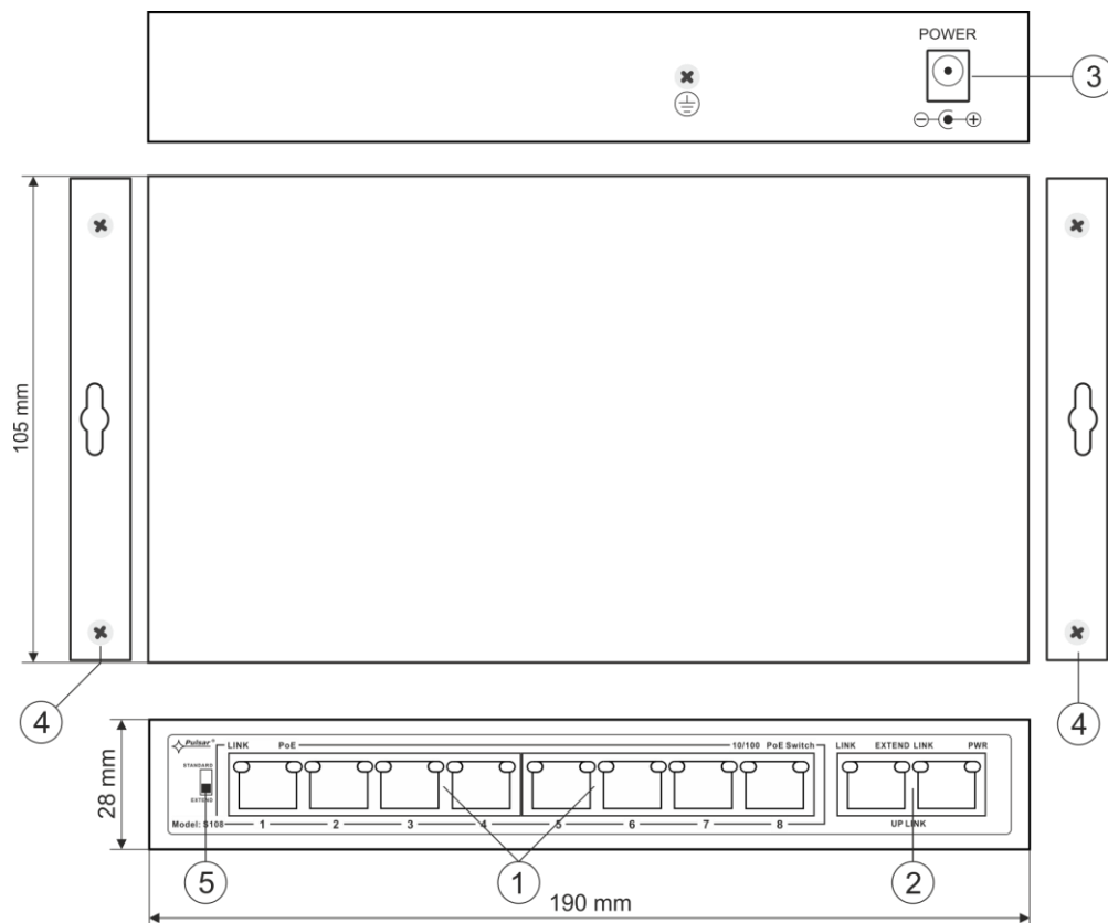
Rys. 2. Widok switch'a.
