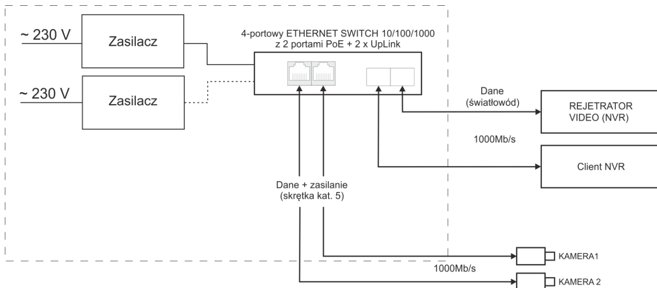
Rys. 1. Schemat blokowy.
