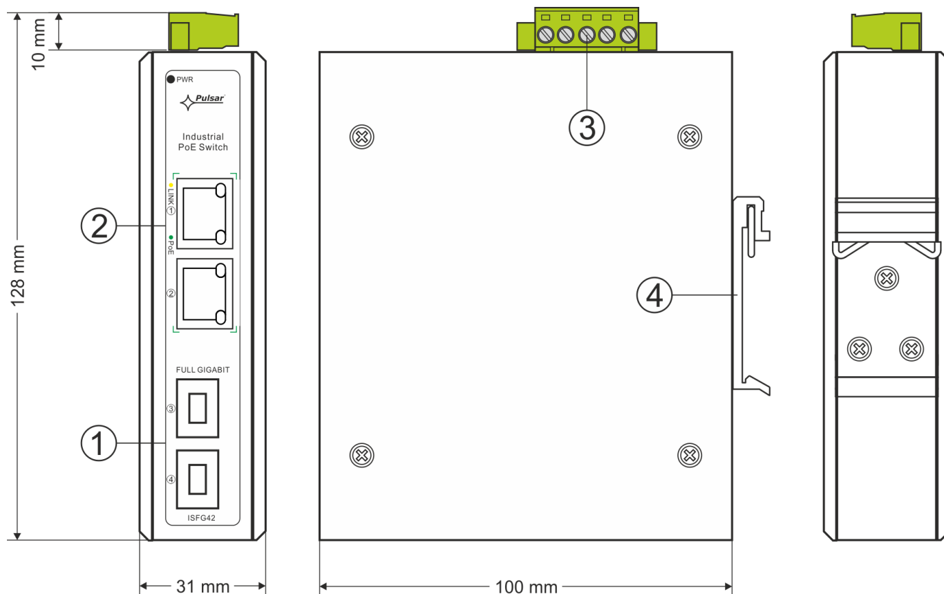
Rys. 2. Widok switch'a.
