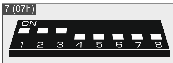
Rys. 6. Sposób ustawienia przełączników DIP-switch w ekspanderze INT-RX-S.
