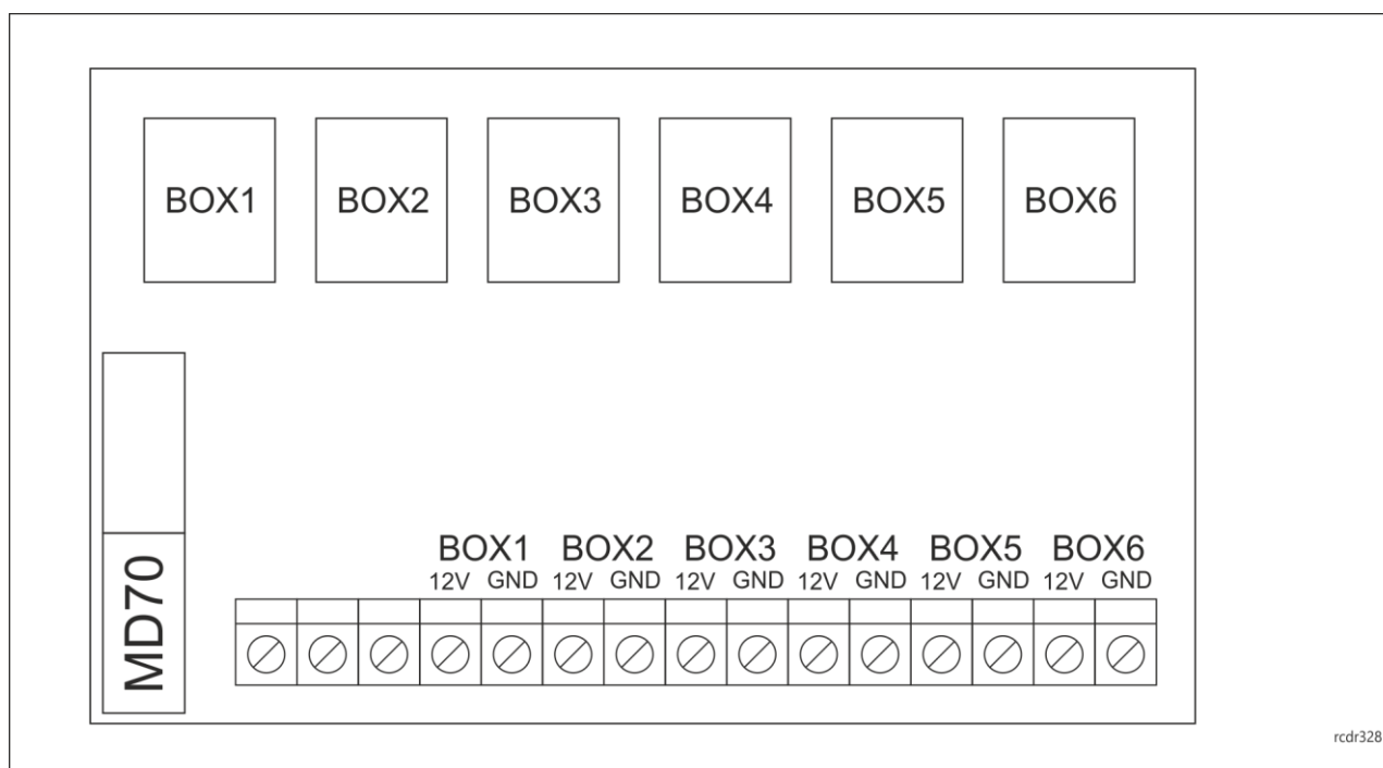
Rys. 11 Moduł podłączeniowy w obudowie panelu kontrolnego
