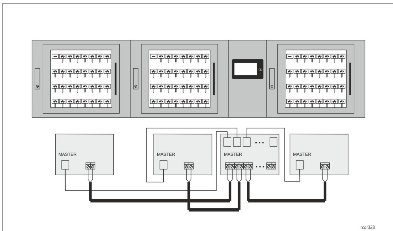
Rys. 10 Podłączenie dodatkowych szaf (RKD32EXT) do depozytora (RKD32)
