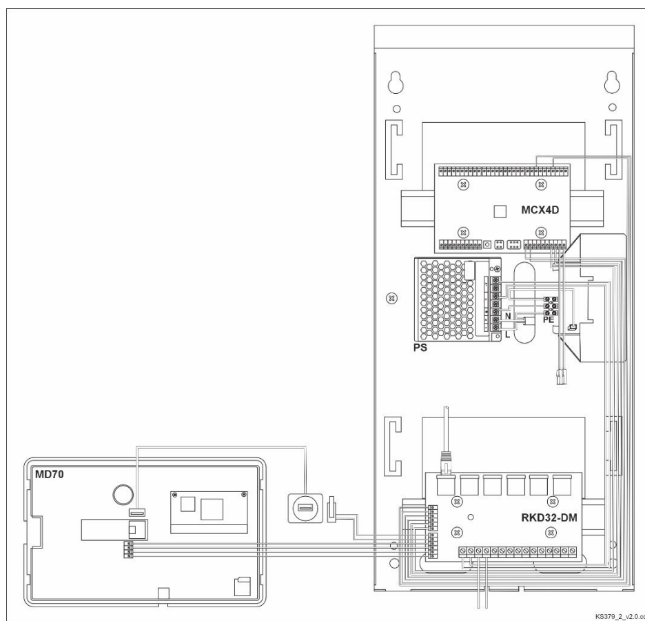
Rys. 7 Podstawa obudowy panelu kontrolnego
