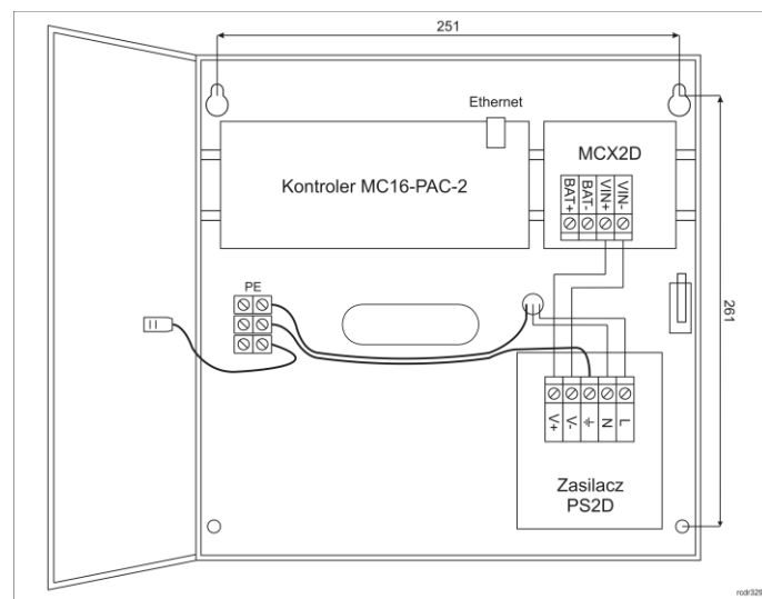
Rys. 1 Zestaw MC16-PAC-2-KIT
