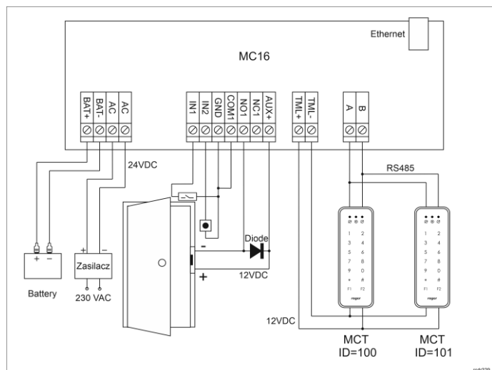
Rys. 2 Typowa obsługa przejścia z czynnikiem serii MCT
