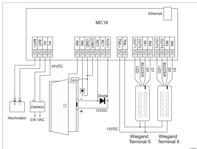
Rys. 3 Typowa obsługa przejścia z czynnikiem Wiegand
