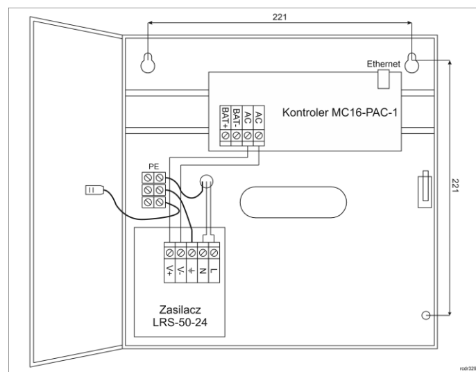
Rys. 1 Zestaw MC16-PAC-1-KIT
