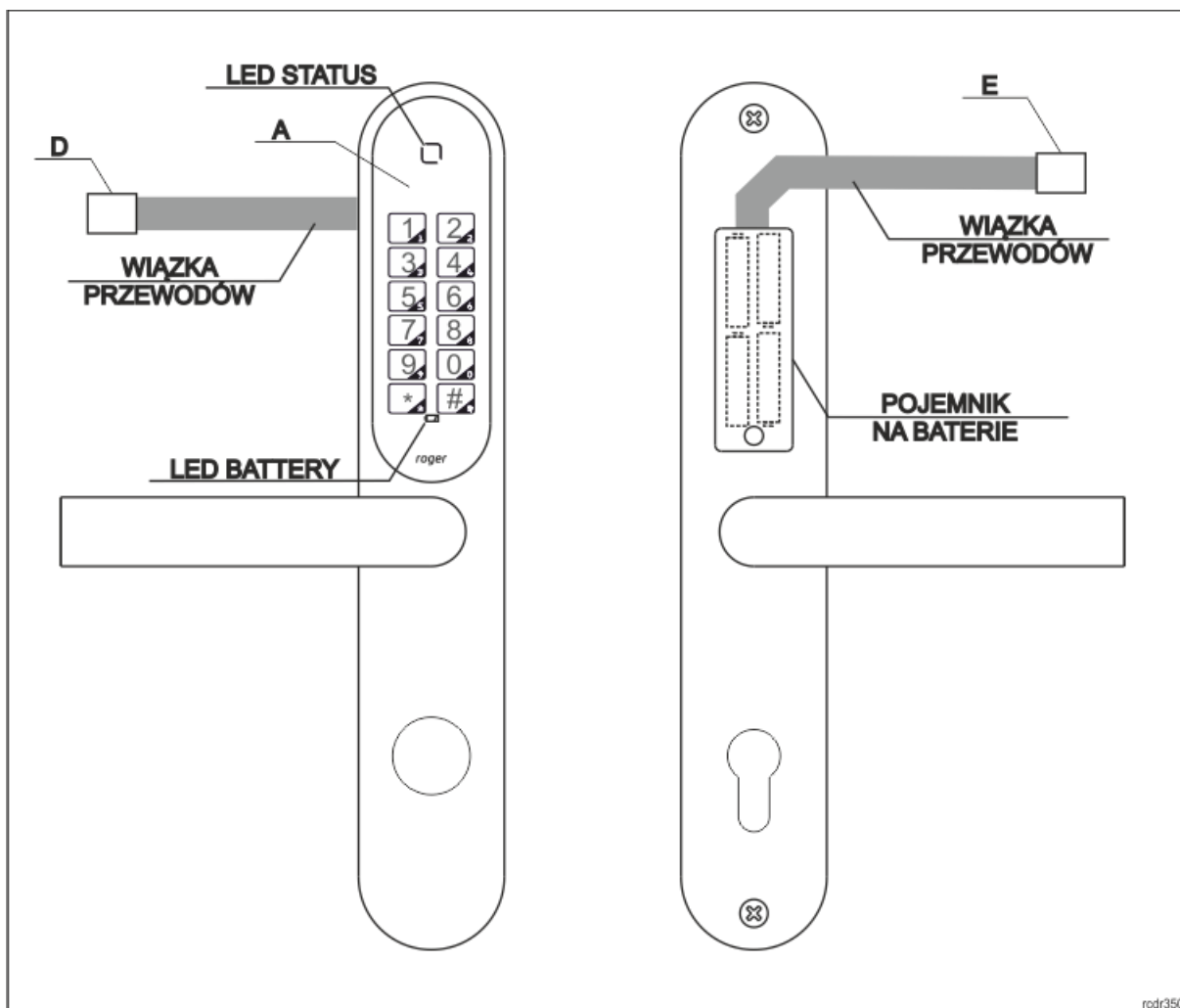
Rys. 3. Widok szyldów
