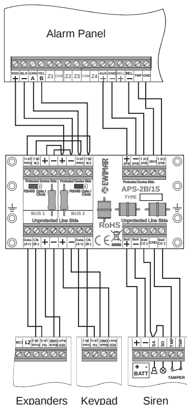
Ochrona 8 linii alarmowych czujek wewnętrznych z separacją zasilania
