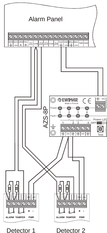
Separacja 8 linii zasilania czujek alarmowych
