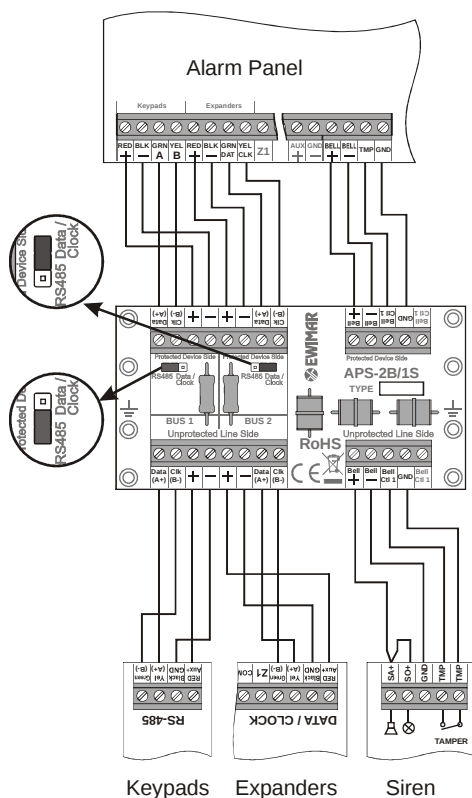
Ochrona 2 magistral i sygnalizatora bez własnego zasilania
