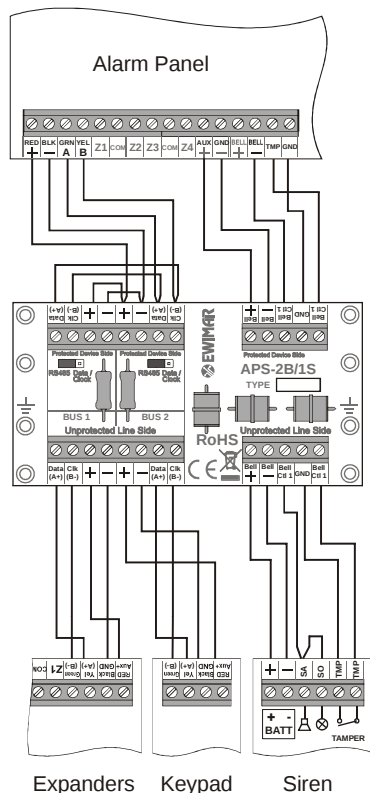
Ochrona 8 linii alarmowych czujek wewnętrznych i wspólnego zasilania
